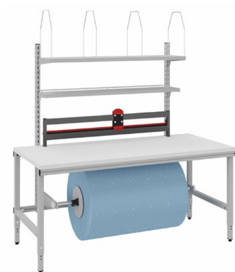
Verpackungstisch OK-V1
